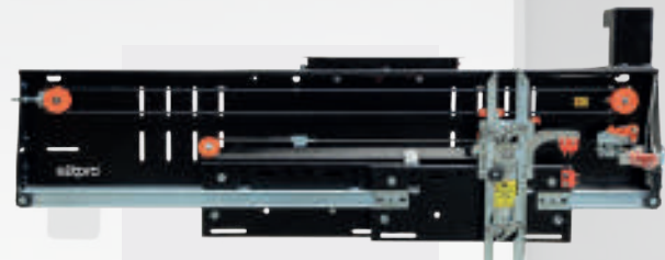
Automatic Telescopic Door
